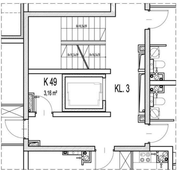
RZUT PIĘTRA II
