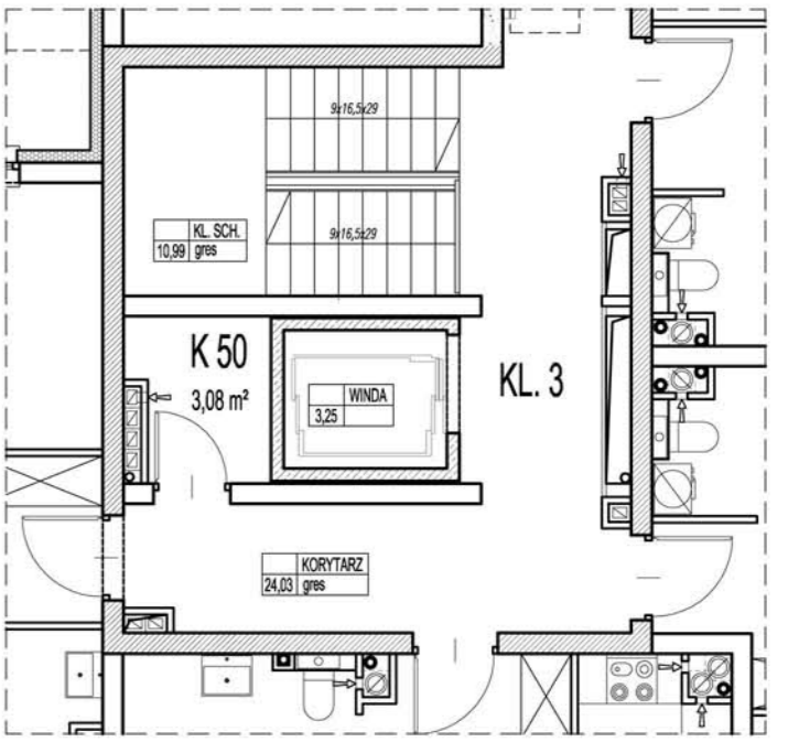
RZUT PIĘTRA III
