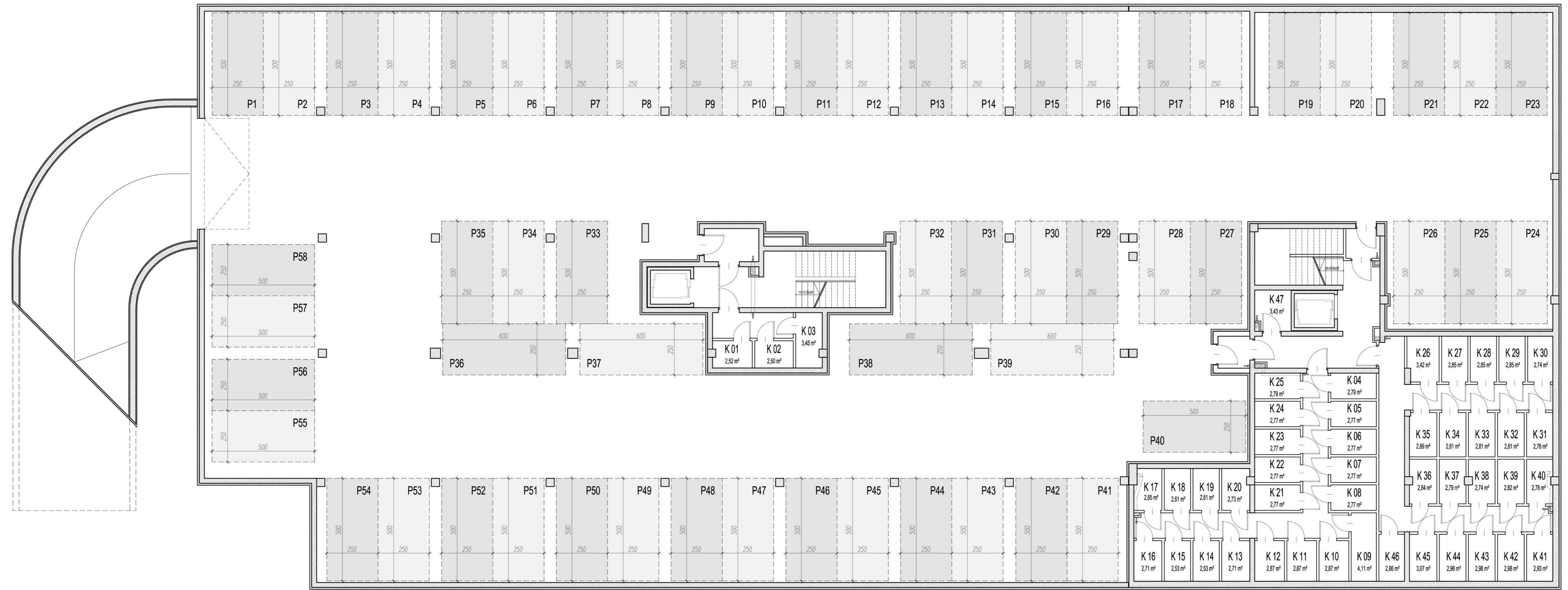
RZUT PIWNIC
